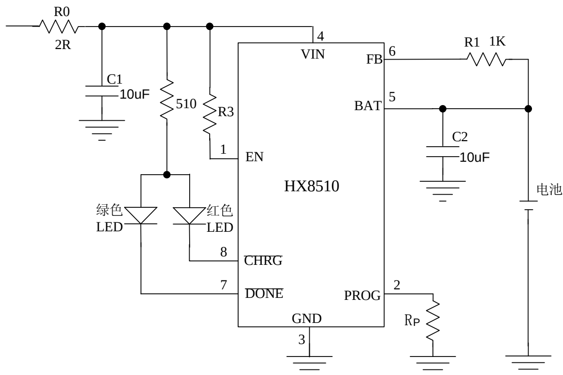
图 1 应用电路（单节镍氢电池充电1.2V）
