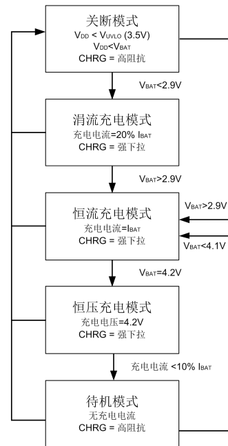
图 3：电池典型充电循环的状态图
