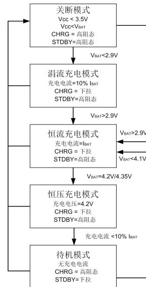
图 3：电池典型充电循环的状态图
