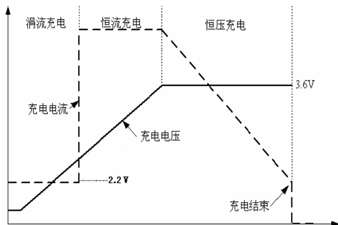
完整的充电循环（1000mAh 电池）
