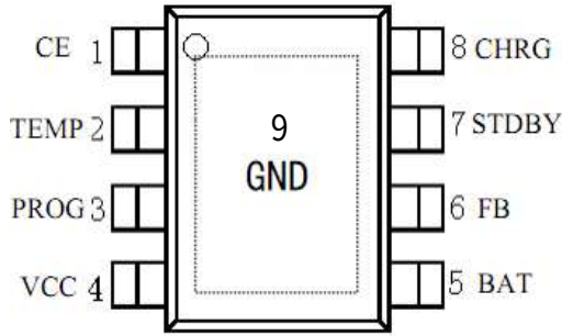
8 引脚 SOP 封装(底部带有散热片)
