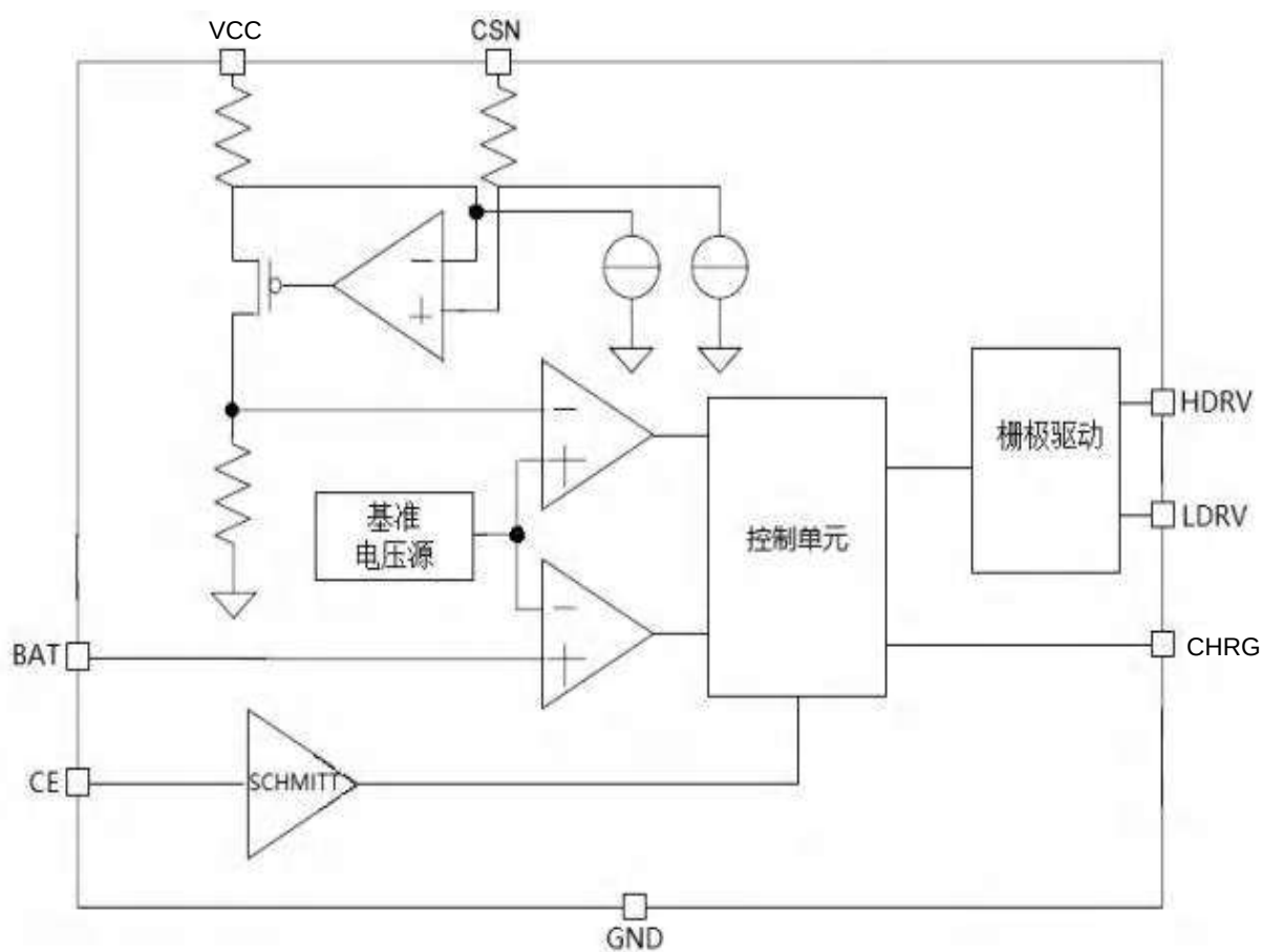
图 3 功能框图
